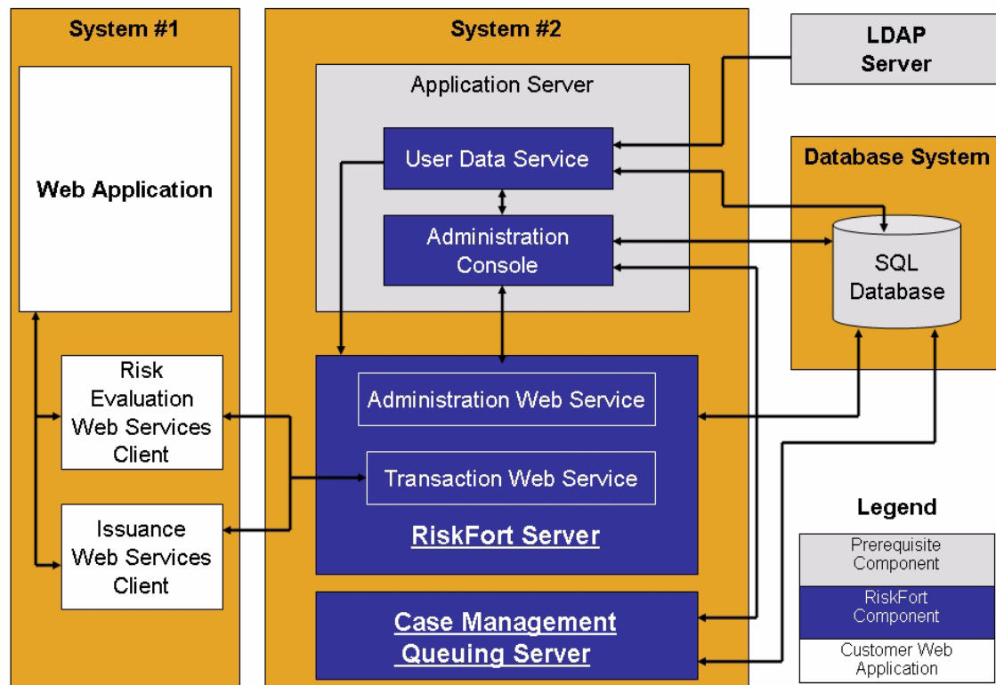
図 2-5 分散システム上の RiskFort（単一アプリケーションとしての Web サービス）
