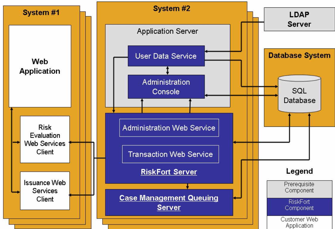
図 2-8 高可用性環境における RiskFort (Web サービス)
