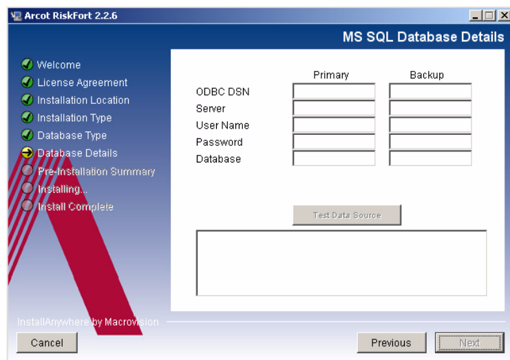
図 4-4 [MS SQL Database Details] 画面
