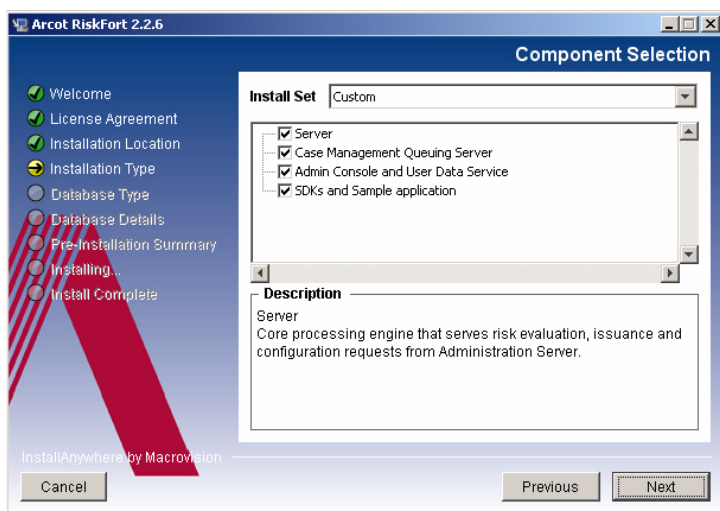
図 5-3 [Component Selection] 画面
