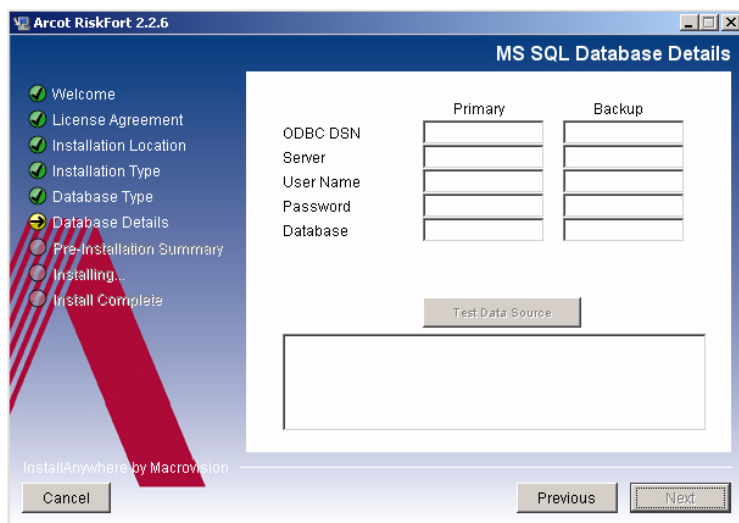
図 5-5 [MS SQL Database Details] 画面
