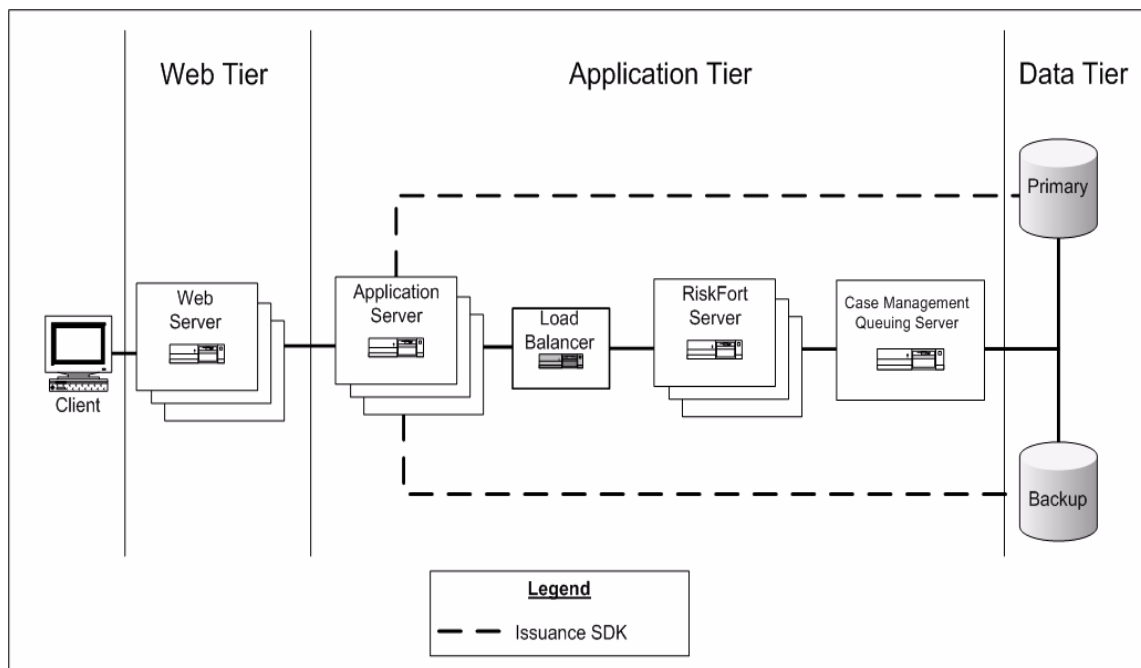
図 2-9 高可用性アーキテクチャ図
