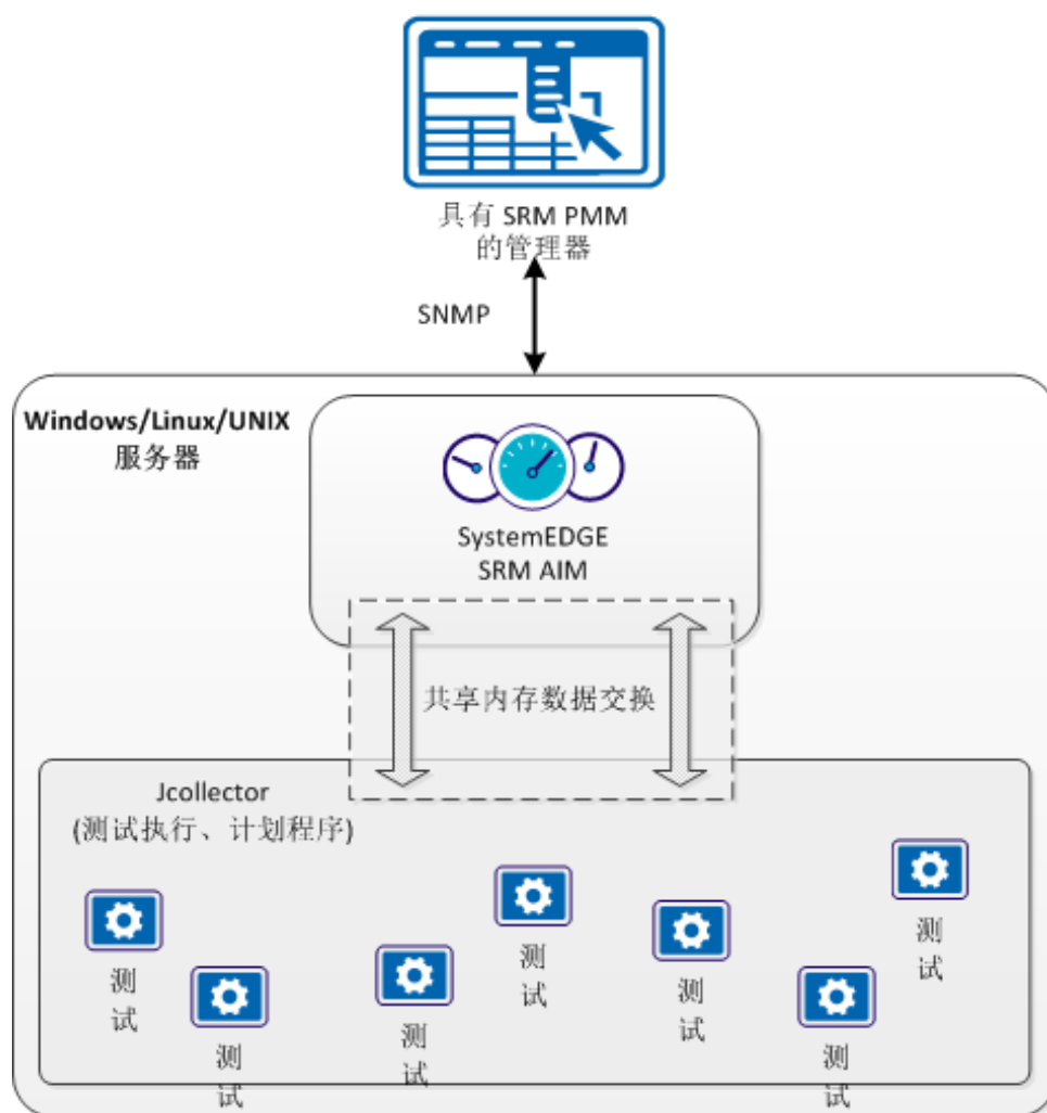
服务响应监控组件之间的交互
