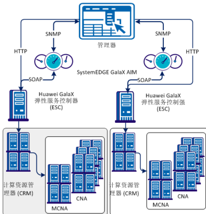
Huawei GalaX 管理组件之间的交互
