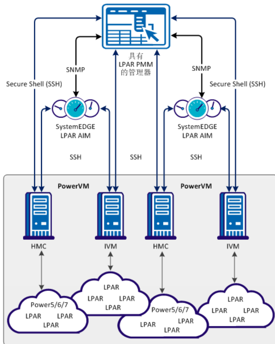
PowerVM 管理组件之间的交互
