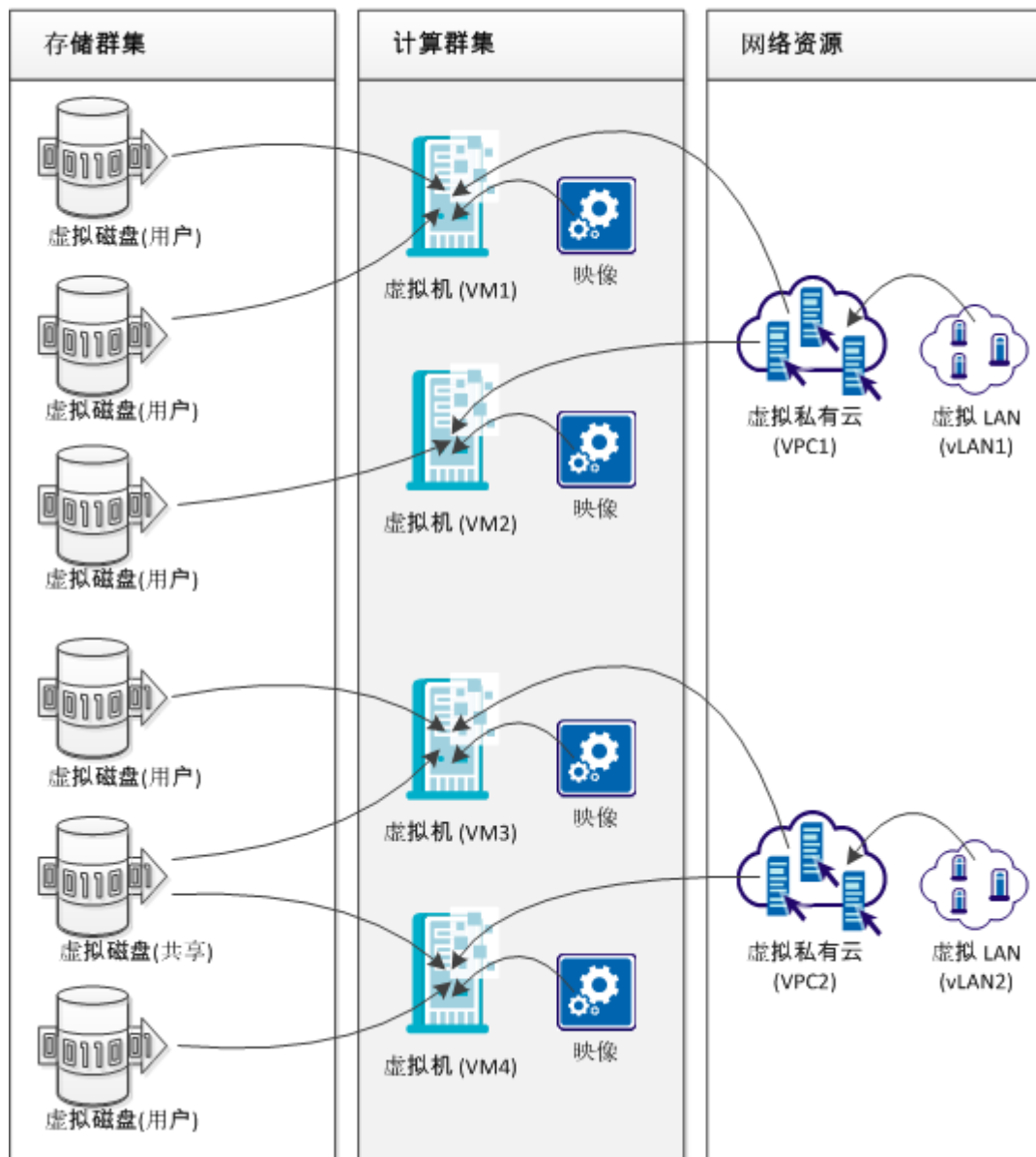
Huawei SingleCLOUD GalaX 组件和它们的关系
