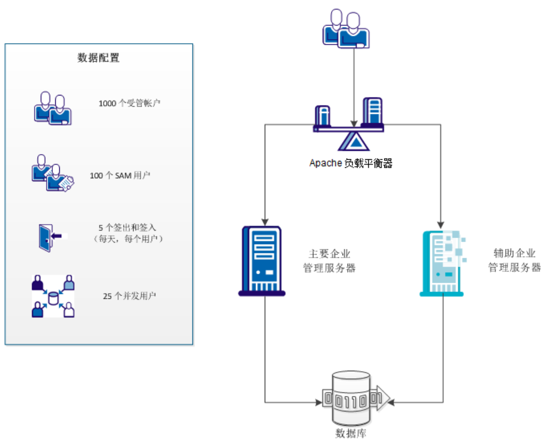
中型环境的部署体系结构 （1000 个受管帐户）
